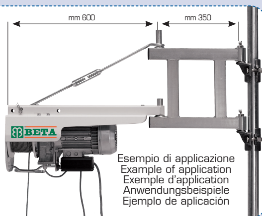
cod. 0007900000 Puntone a finestra Window strut Chevron fenêtre Fensterstütze Puntal a ventana
